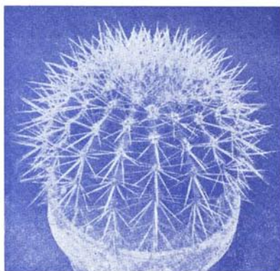
ECHINOCACTUS Grusoni
